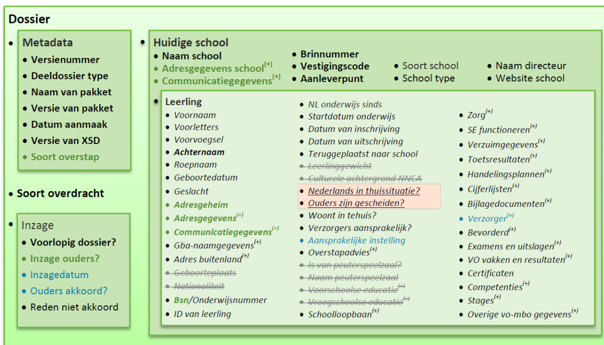
Figuur 16: Overzicht van gegevenselementen in het profiel m.b.t. Dossier.
