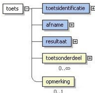
Figuur A.15: Overzicht van toets.
