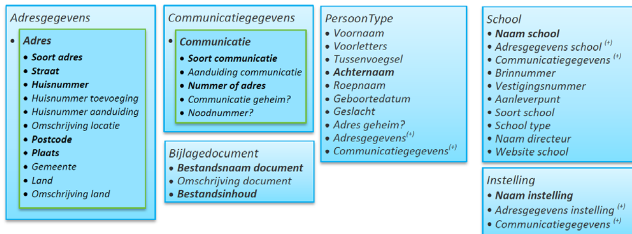
Figuur 8: Schematisch overzicht van de hergebruikte gegevens-elementen binnen Dossier.
