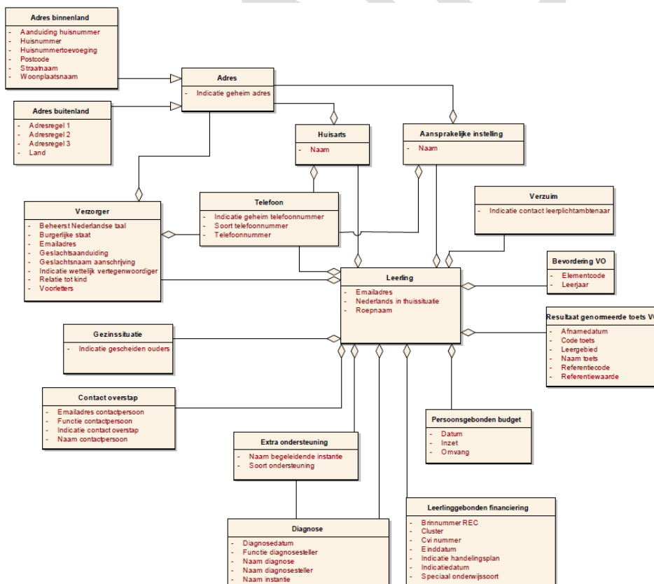
Figuur 15: Overzicht van leerlinggegevens in overstapdossier.
