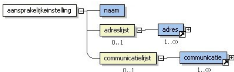
Figuur A.6: Overzicht van aansprakelijkeinstelling.
