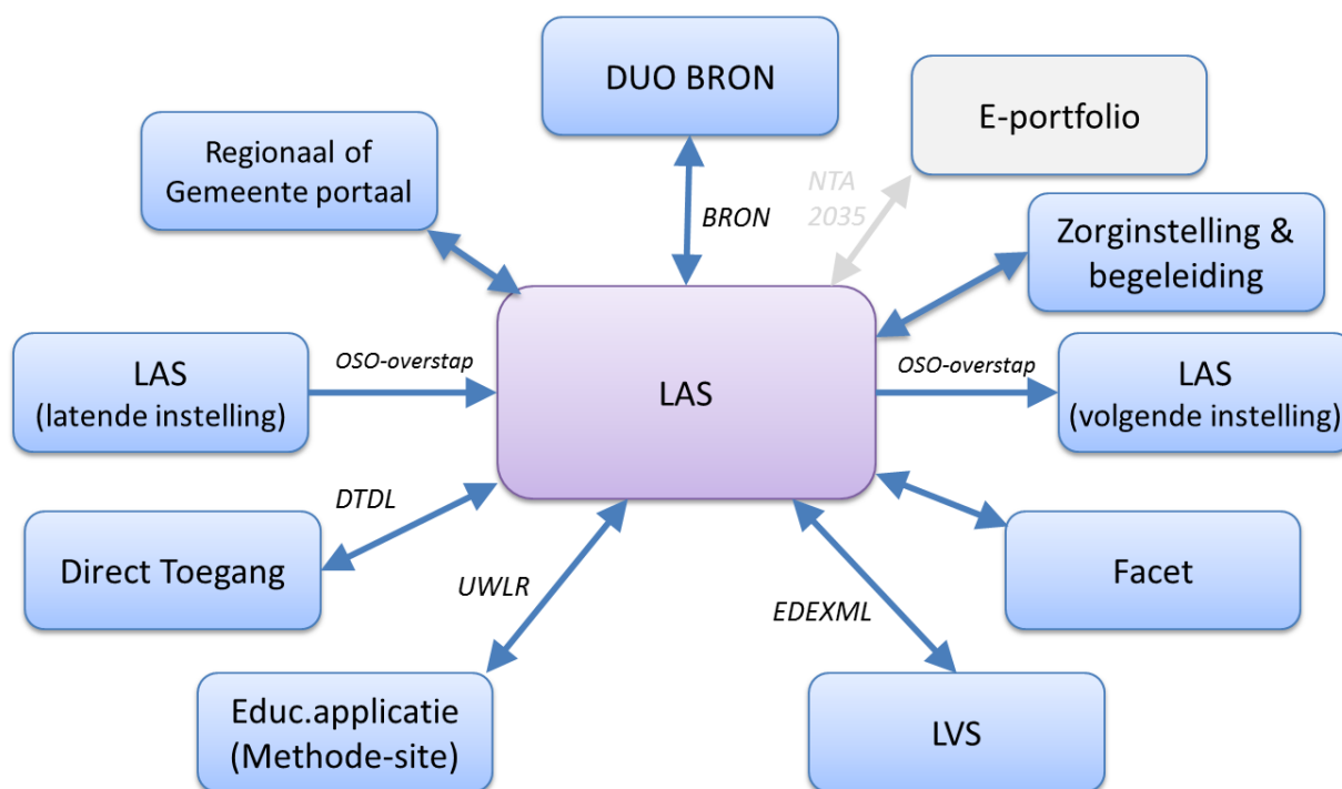
Figuur 4: Uitwisseling van leerlinggegevens van/naar het vo.
