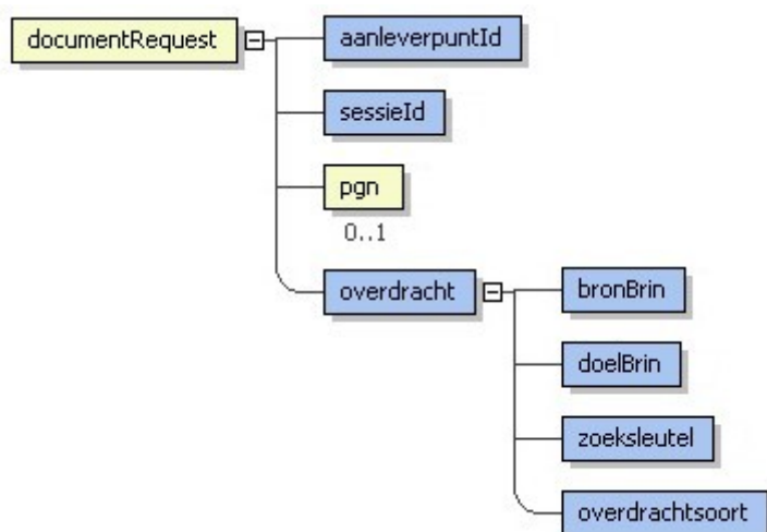
Figuur 13: Overzicht van bericht documentRequest.
