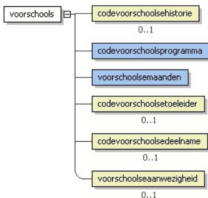
Figuur A.8: Overzicht van voorschools.
