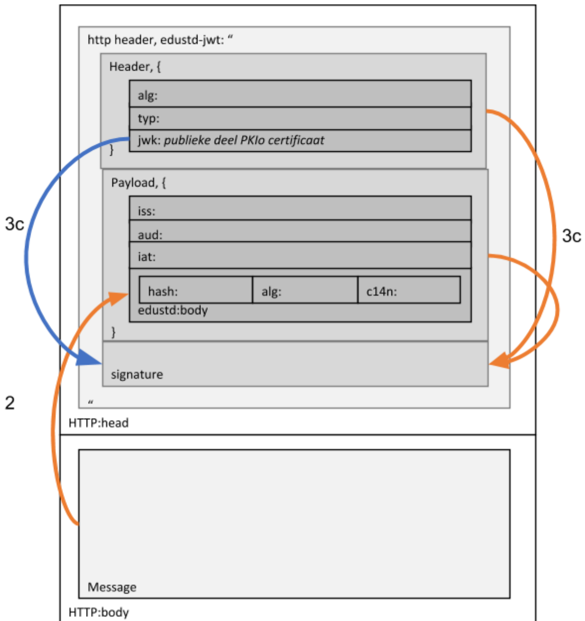
Figuur 3. Structuur van een bericht met JWT ondertekening. De nummers bij de pijlen verwijzen naar acties in Verantwoordelijkheden van afzender .
