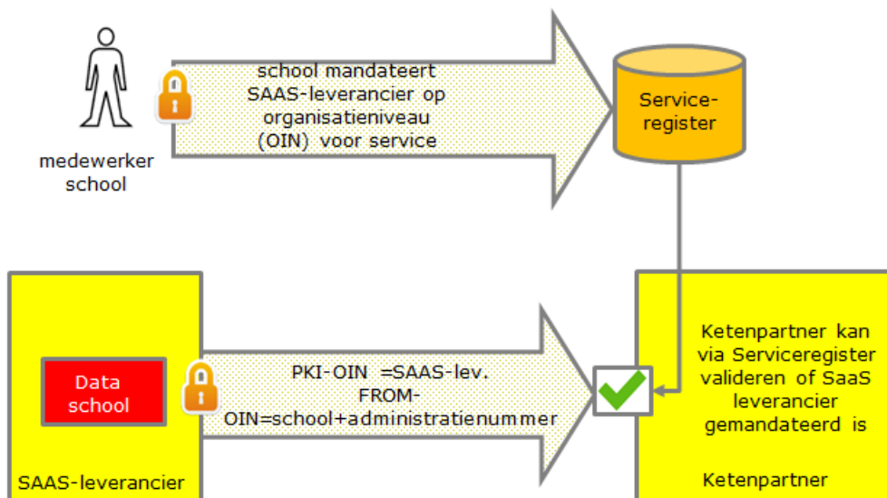
Figuur 4 – SaaS leverancier mandatering bij bevragingen
