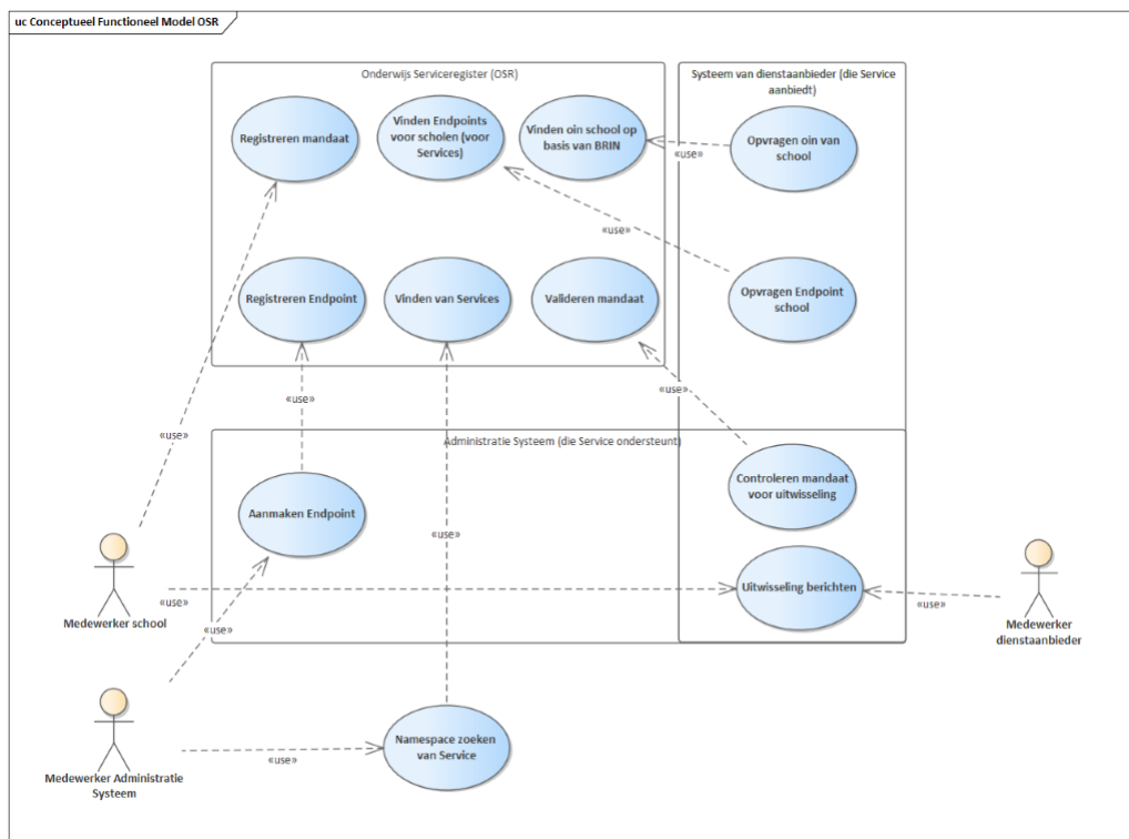
Figuur 15 - Conceptueel functioneel model OSR
