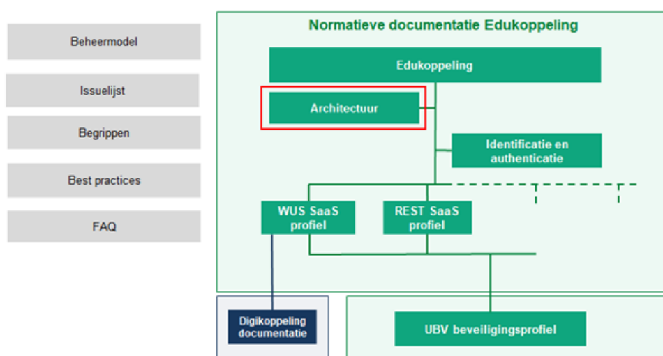
Figuur 1- Positionering van Architectuur binnen Edukoppeling
