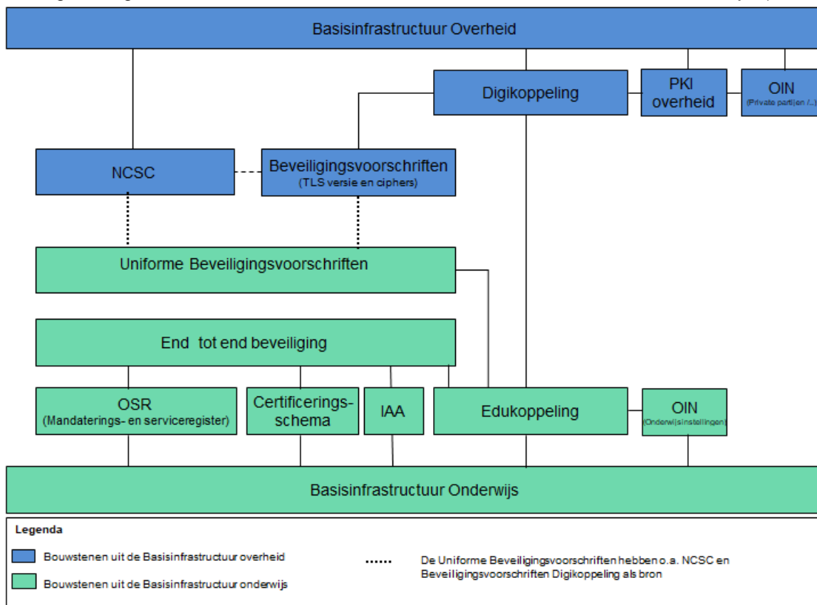
Figuur 14 - Overzicht van bouwstenen om end-to-end beveiliging te realiseren
