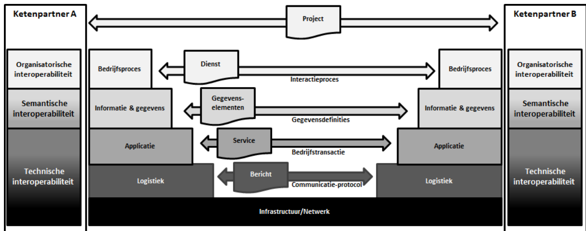
Figuur 3 - Informatie-uitwisselingsmodel - Applicatielaag
