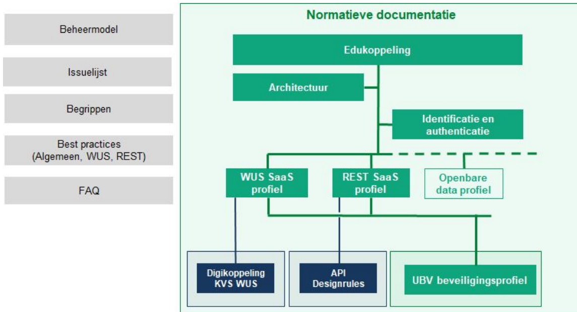
Figuur 2 - Overzicht Edukoppeling documentatie
