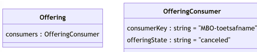
Figuur 2.10: Offering gegevensmodel t.b.v. Zitting verwijderen in 2. Zittingsplan
