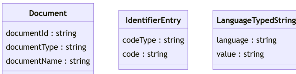
Figuur 4.0.A: Algemene gegevensobjecten in het gegevensmodel
