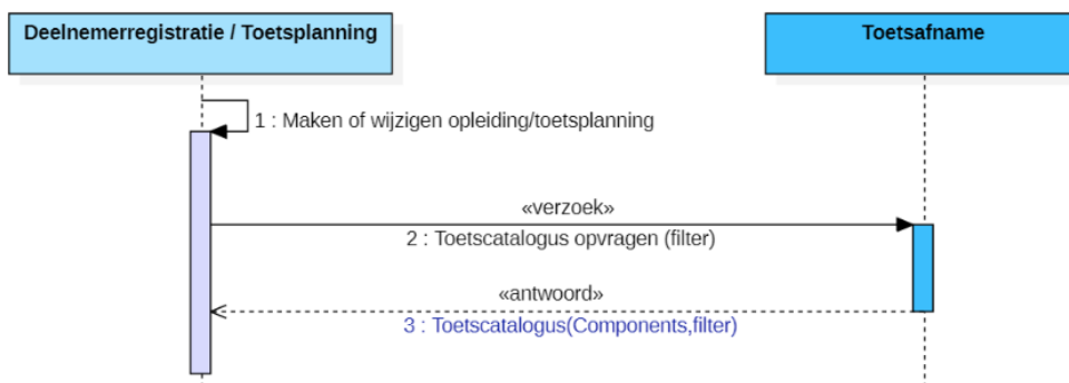
Figuur 0.2: Toetscatalogus opvragen interactiemodel
