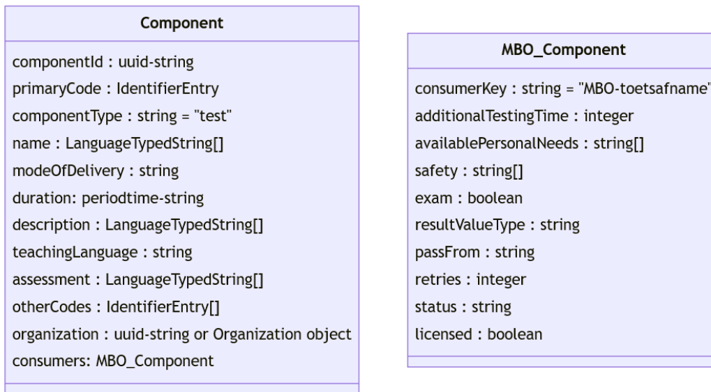
Figuur 4.2.A: Component gegevensmodel
