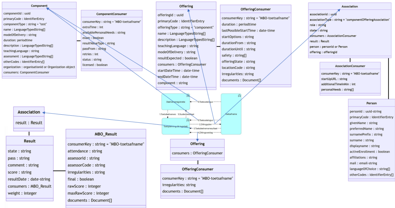
Figuur 4.0.A: Gegevensobjecten per informatiestroom (informatiestromen 0, 2 t/m 4)
