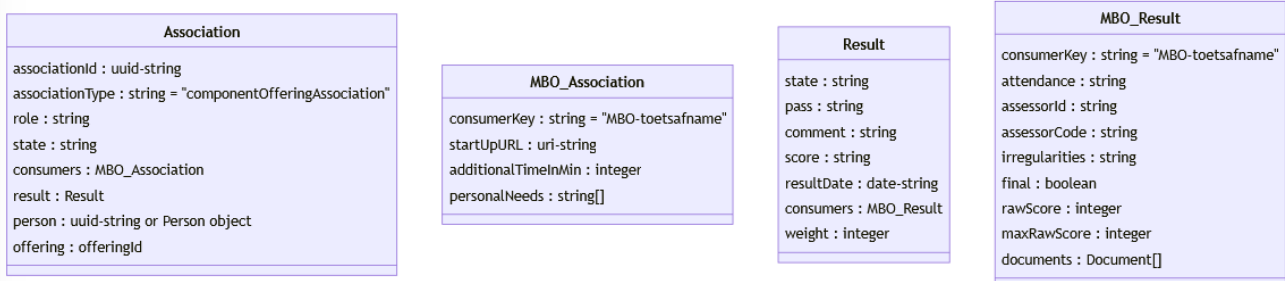
Figuur 3.8: Association gegevensmodel t.b.v. Deelname(s) ophalen voor Toetsdeelnemerresultaat
