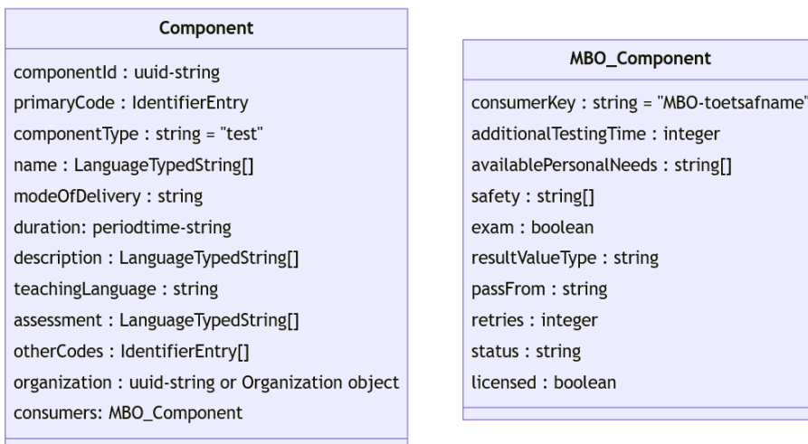
Figuur 0.5: Component gegevensmodel
