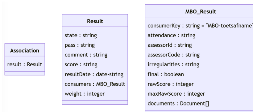
Figuur 3.6: Association gegevensmodel t.b.v. aanwezigheidsresultaat (links) en scoreresultaat (rechts)
