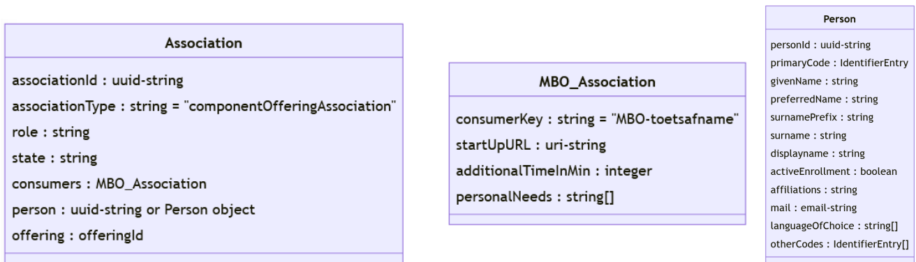
Figuur 2.7: Association gegevensmodel t.b.v. 2. Zittingsplan
