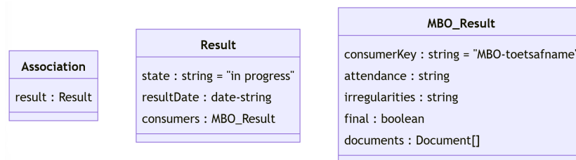
Figuur 3.5: Association gegevensmodel t.b.v. aanwezigheidsresultaat
