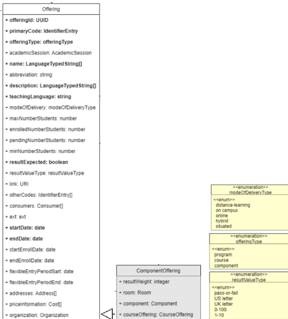
Figuur 6.1.D: OOAPI gegevensobject Offering (ComponentOffering is uitbreiding Offering) voor Zitting
