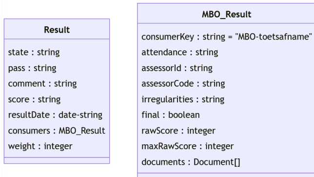
Figuur 4.1.B: Result gegevensmodel
