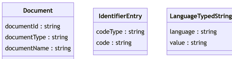
Figuur 4.0.B: Algemene gegevensobjecten in het gegevensmodel
