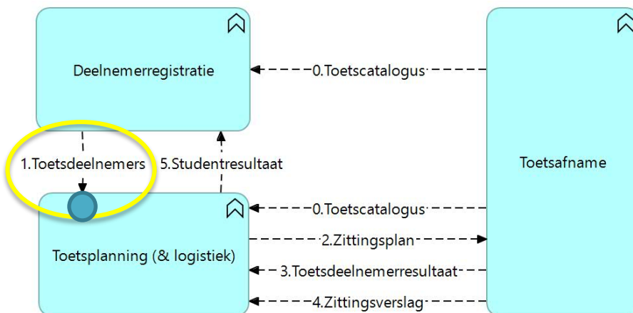
Figuur 1.3: Koppelvlak bij Toetsplanning voor Toetsdeelnemers
