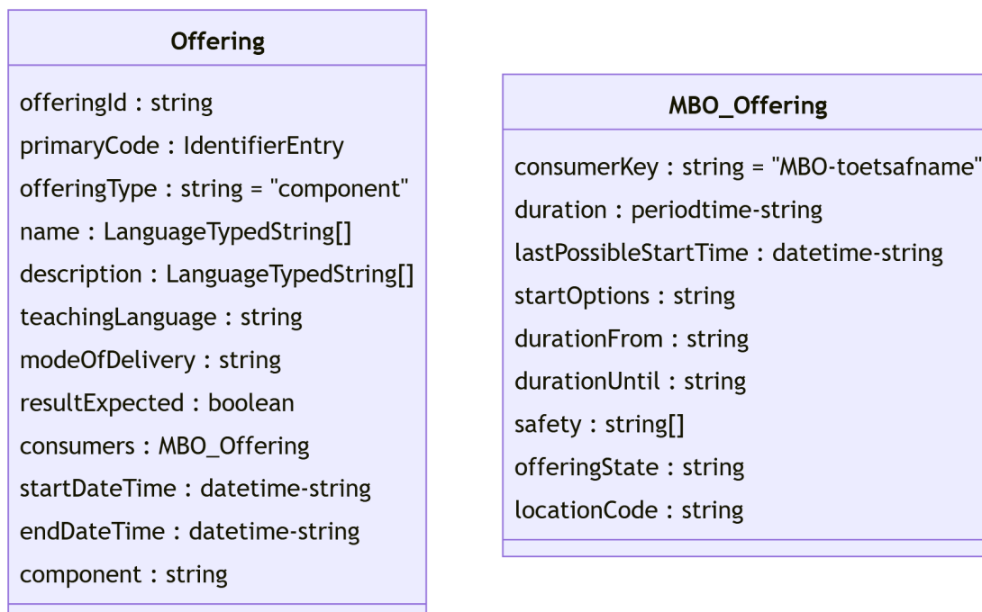
Figuur 2.9: Offering t.b.v. gegevensmodel t.b.v. 2. Zittingsplan
