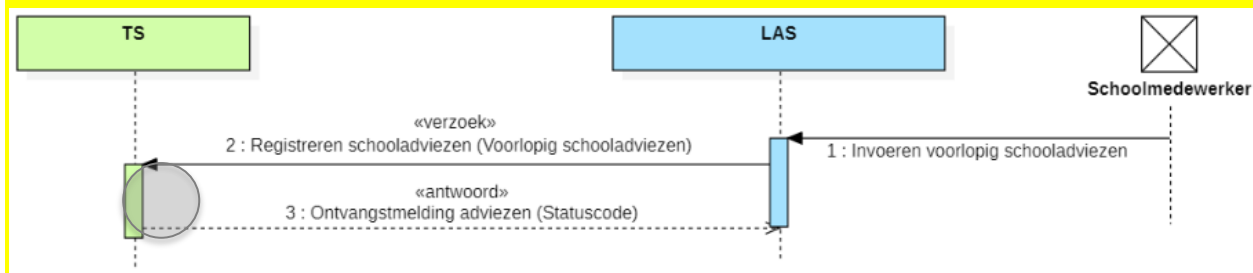
Figuur 13: Interactie “Voorlopig schooladviezen”
