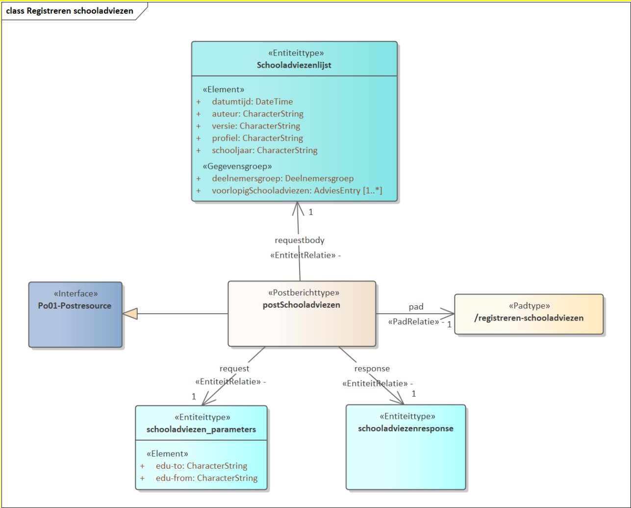
Figuur 15: BSM van het bericht “Registreren schooladviezen”
