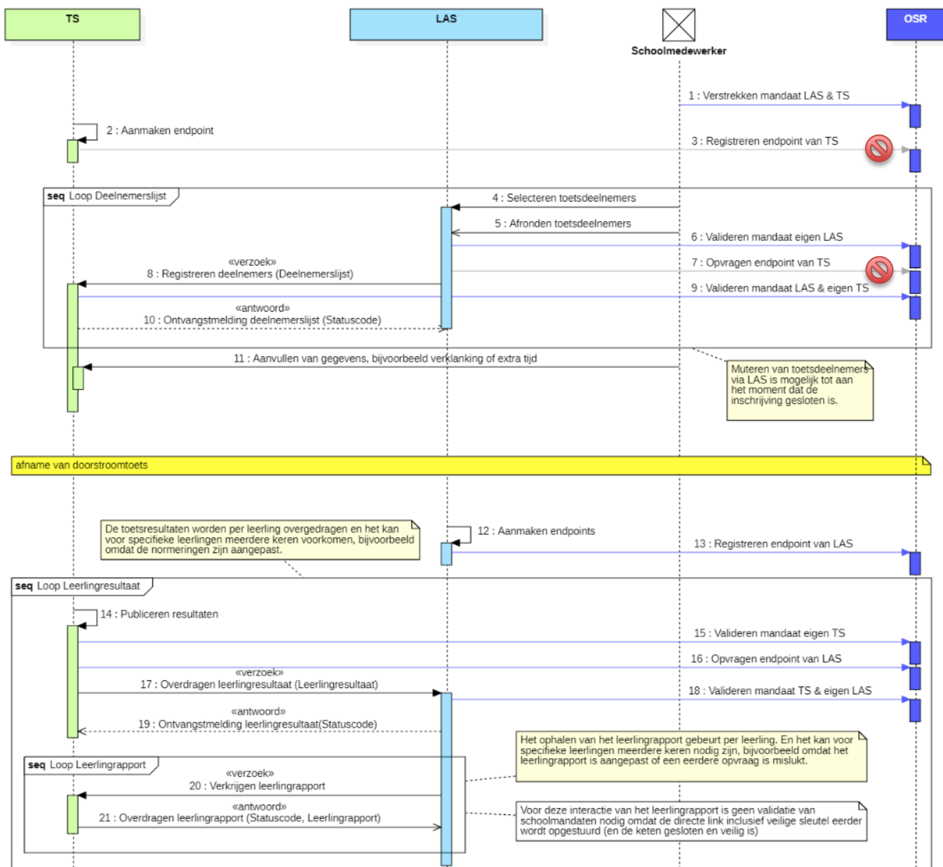
Figuur 23: Interactieschema Toetsdeelnemers en Toetsresultaten, inclusief interacties met het OSR
