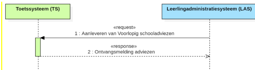
Figuur 5: Transactiepatroon “Push” t.b.v. uitwisseling “Voorlopig schooladviezen”
