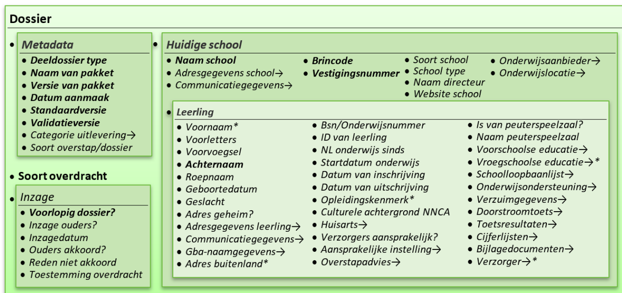
Figuur 5: Overzicht van gegevenselement Dossier.
