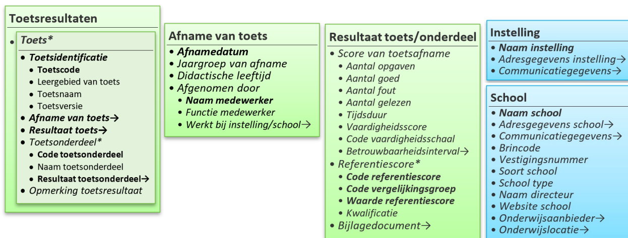
Figuur A.18: Overzicht van gegevensblok Toetsresultaten en deelelementen.
