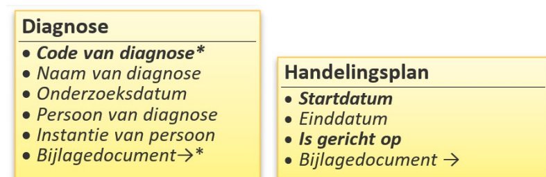
Figuur A.12: Overzicht van gegevensblokken Diagnose en Handelingsplan.
