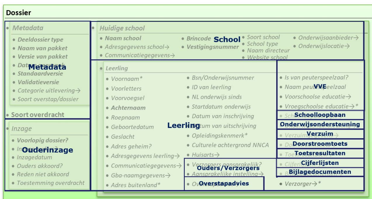
Figuur 13: Categorieën van Dossier in OSO Gegevensset.
