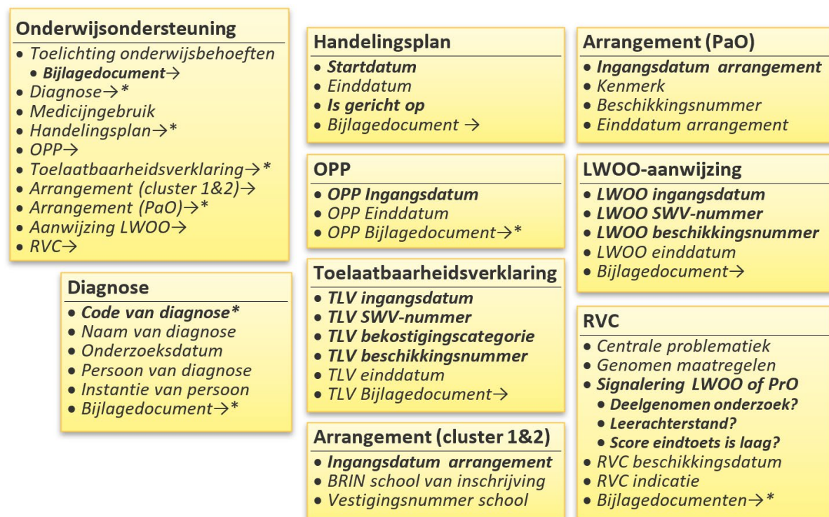
Figuur: Onderwijsondersteuning gegevensmodel
