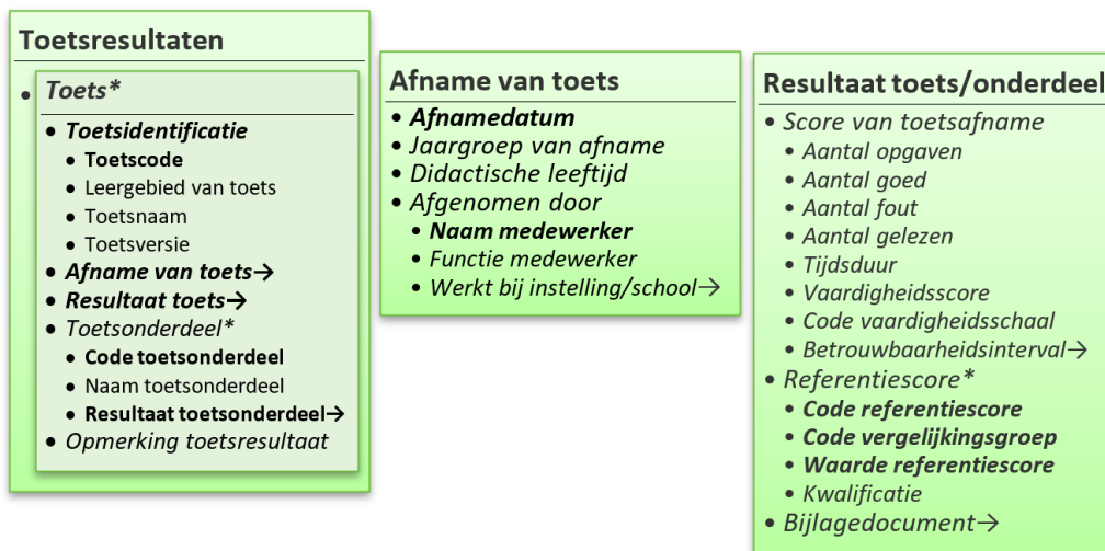
Figuur: Toetsresultaten gegevensmodel
