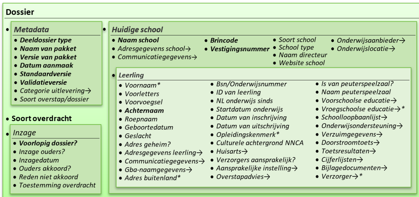
Figuur: Dossier gegevensmodel
