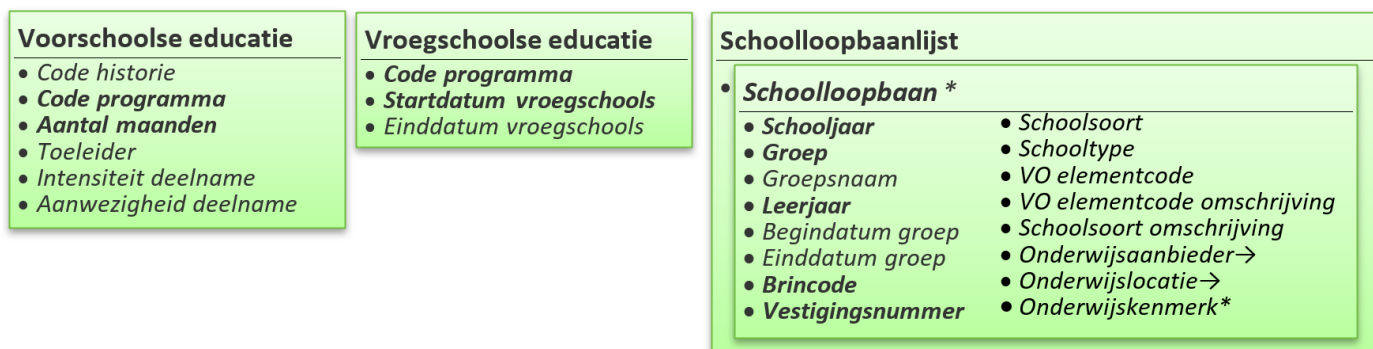
Figuur: Voorschoolse en Vroegschoolse Educatie (VVE) & Schoolloopbaan gegevensmodel
