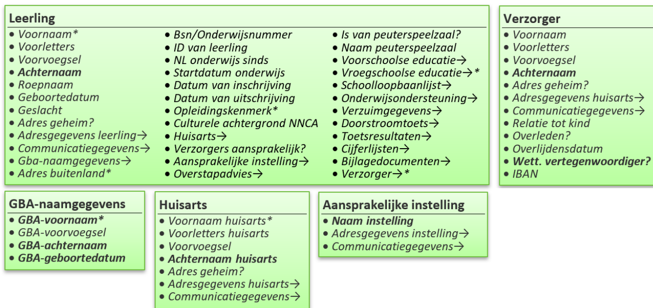
Figuur: Leerling & Verzorger gegevensmodel
